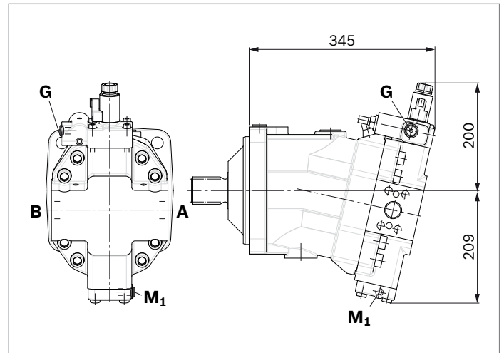
▼ EP5D1, EP6D1 – Proportionalverstellung elektrisch, negative Kennung, mit Druckregelung fest eingestellt
