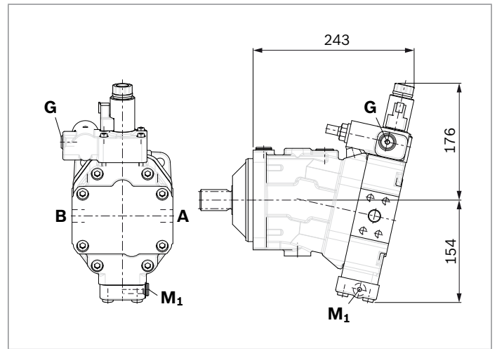
▼ EP5D1, EP6D1 – Proportionalverstellung elektrisch, negative Kennnung, mit Druckregelung fest eingestellt
